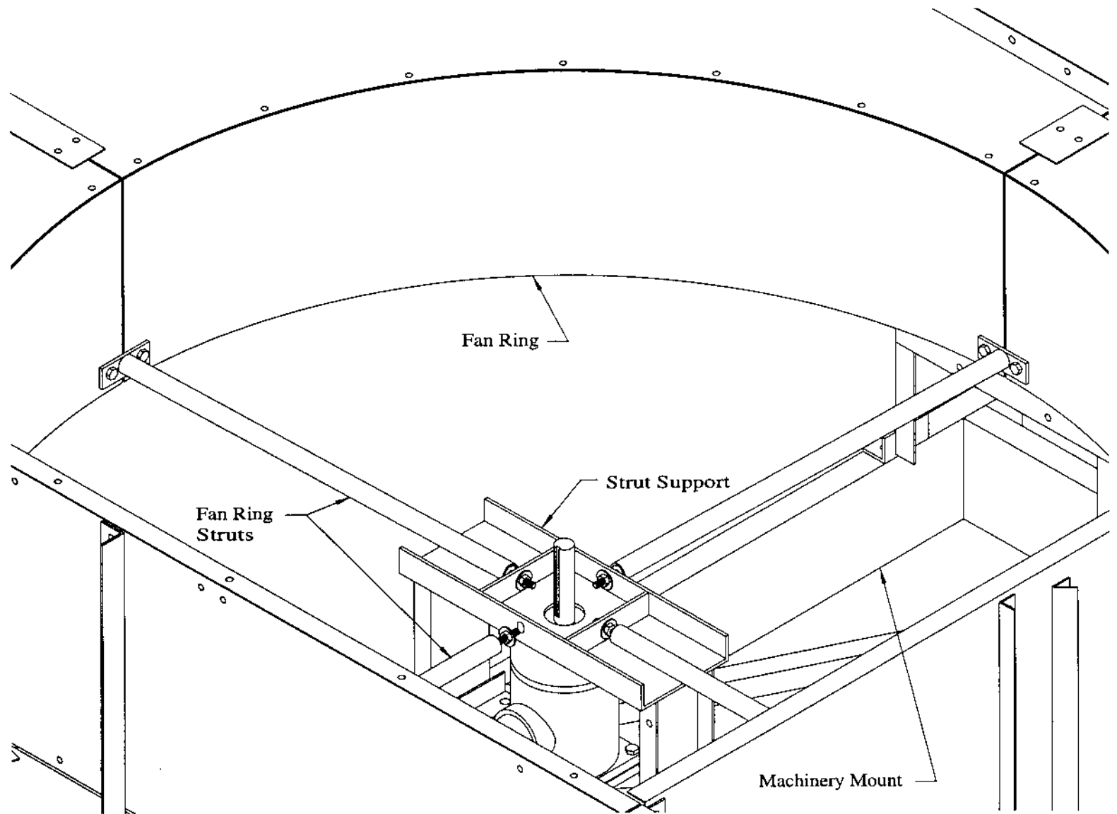
FIG. C5 - FAN RING STRUTS
