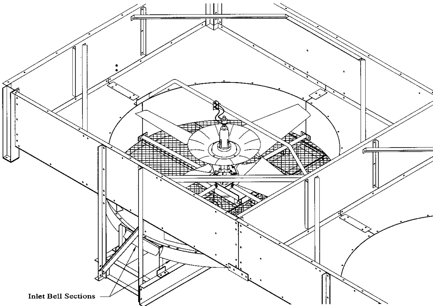
FIG. D2 - INLET BELL
