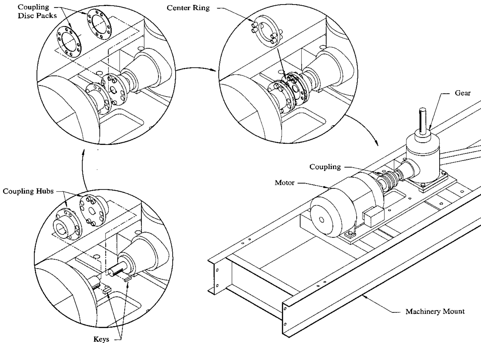
FIG. C2 - COUPLING
